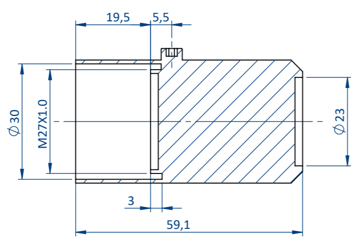
COUPE A-A
