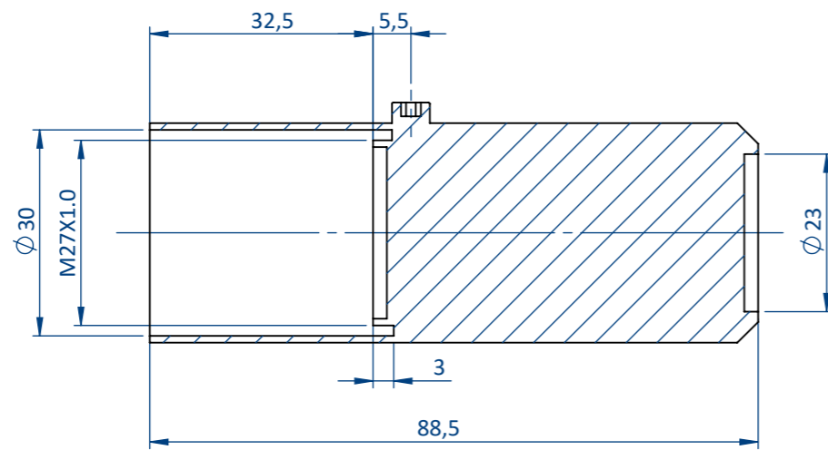
COUPE A-A
